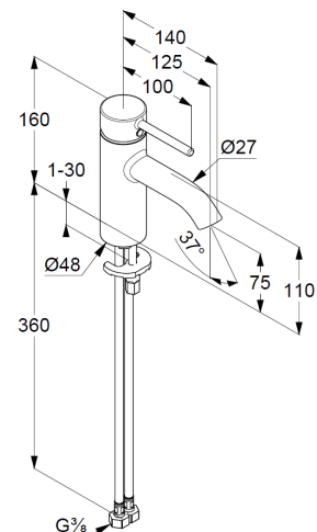
Maßzeichnung
