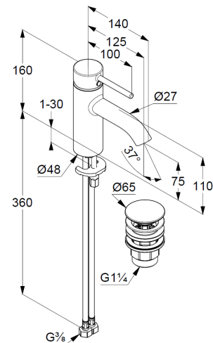
Maßzeichnung
