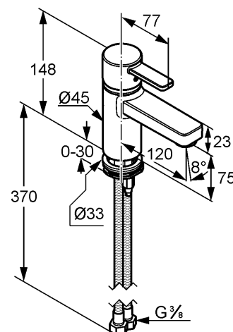
Maßzeichnung
