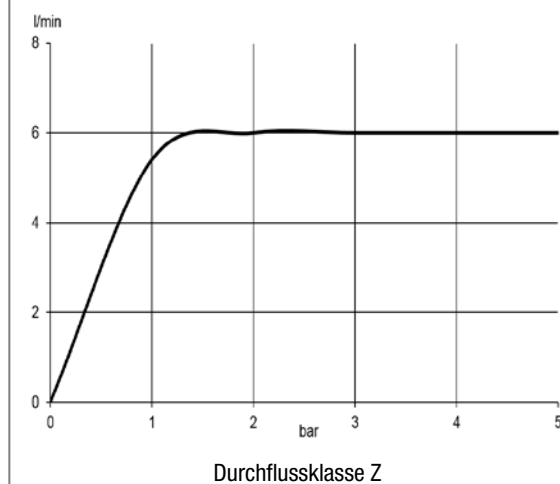
Durchflussdiagramm
