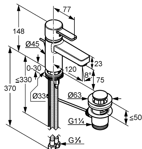
Maßzeichnung
