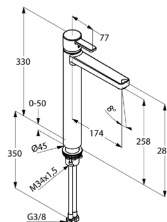
Maßzeichnung
