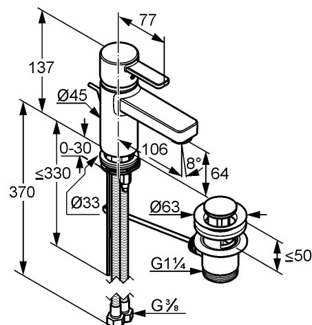
Maßzeichnung
