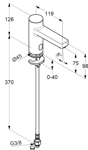
Maßzeichnung
