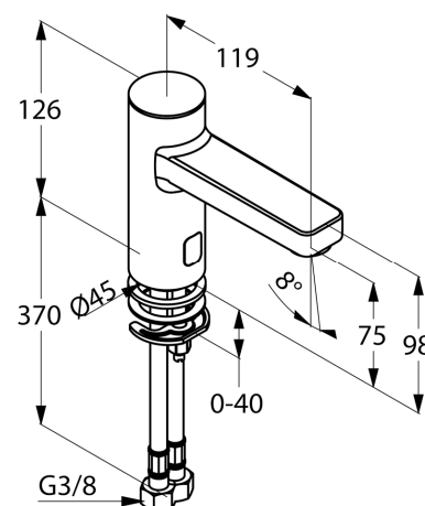
Maßzeichnung
