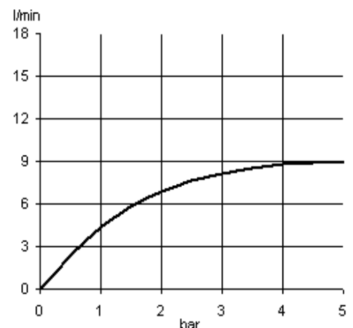
Durchflussdiagramm
