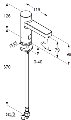
Maßzeichnung
