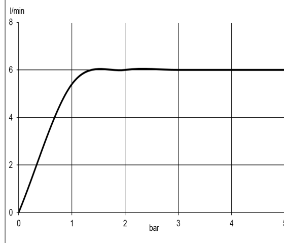
Durchflussdiagramm
