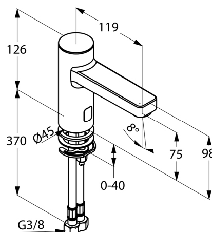
Maßzeichnung
