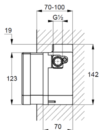
Maßzeichnung
