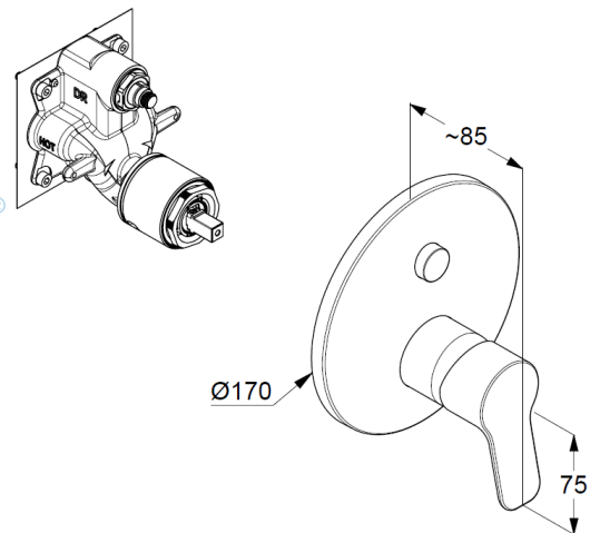
Maßzeichnung
