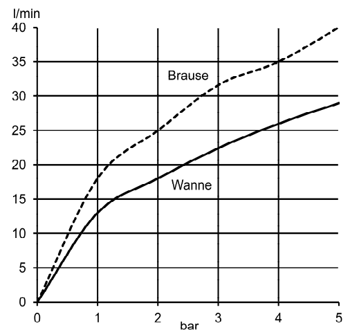
Durchflussdiagramm
