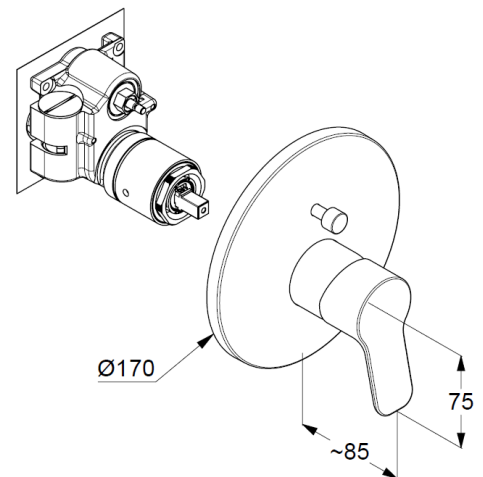
Maßzeichnung
