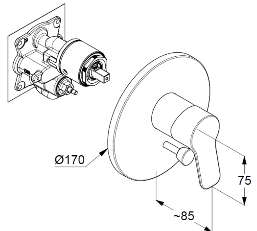
Maßzeichnung
