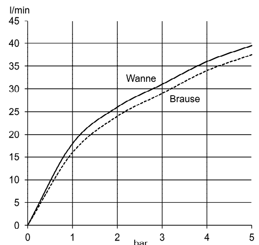
Durchflussdiagramm
