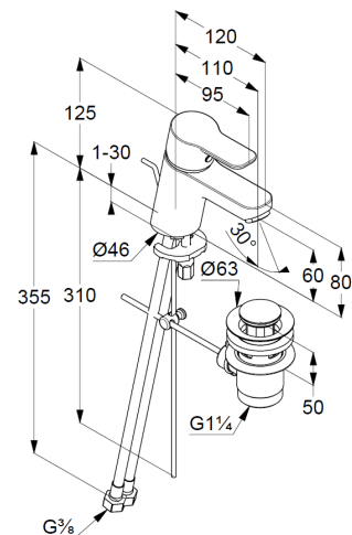
Maßzeichnung
