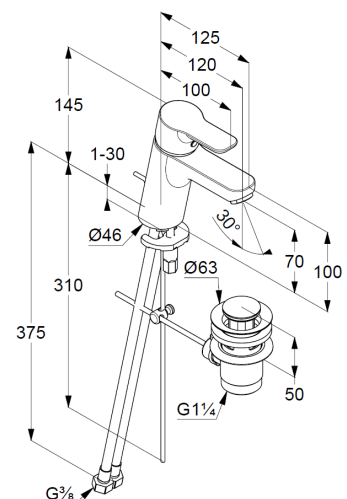
Maßzeichnung
