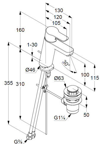
Maßzeichnung
