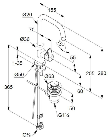
Maßzeichnung
