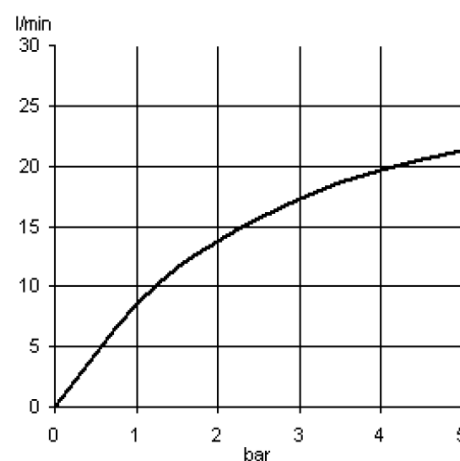
Durchflussdiagramm
