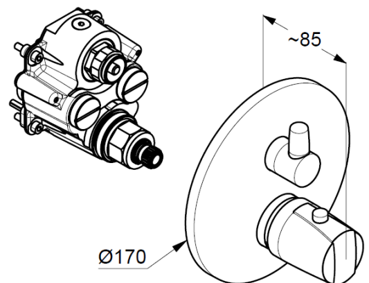
Maßzeichnung
