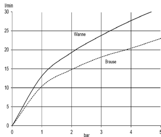
Durchflussdiagramm
