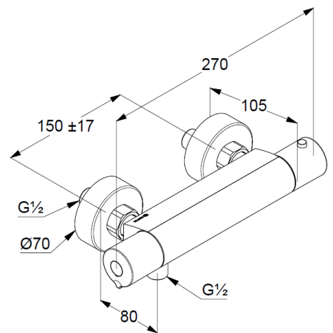
Maßzeichnung
