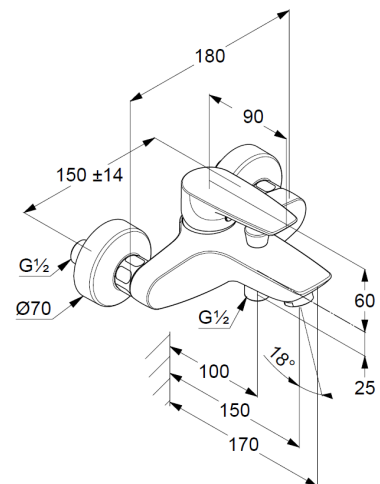
Maßzeichnung
