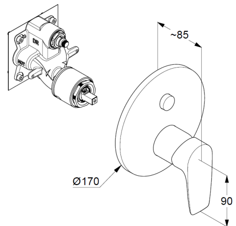
Maßzeichnung
