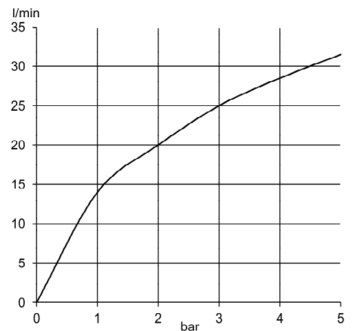
Durchflusssdiagramm
