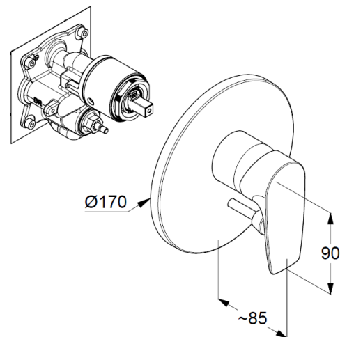
Maßzeichnung
