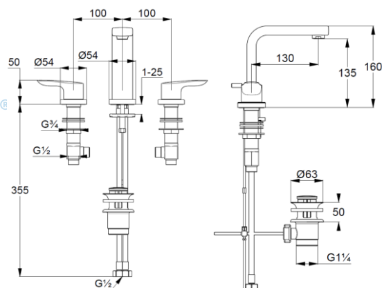
Maßzeichnung
