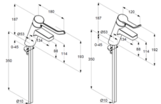
Maßzeichnung
