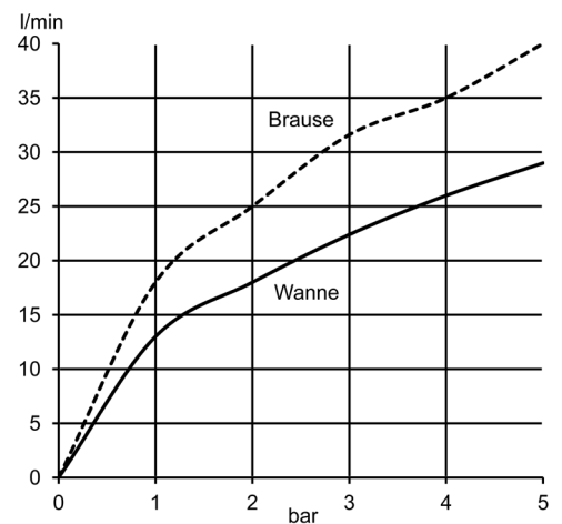
Durchflussdiagramm
