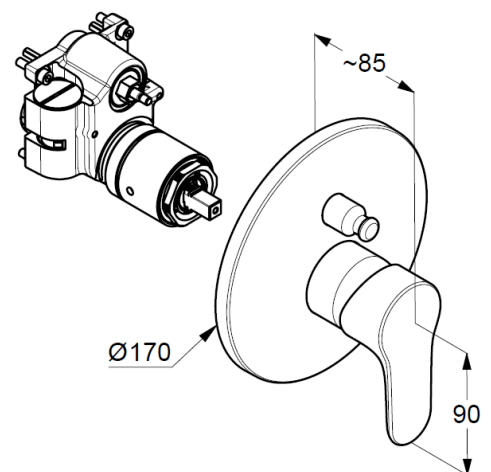
Maßzeichnung
