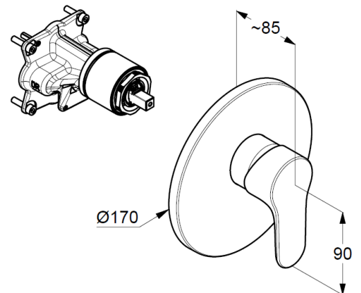
Maßzeichnung
