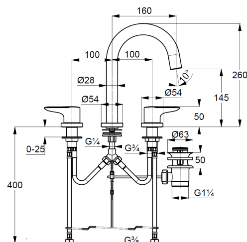
Maßzeichnung
