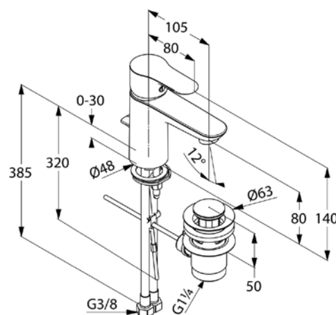
Maßzeichnung
