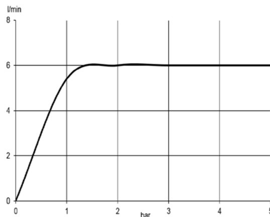
Durchflussdiagramm
