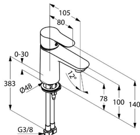
Maßzeichnung
