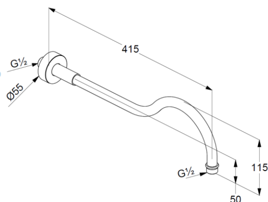
Maßzeichnung
