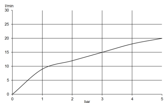
Durchflussdiagramm
