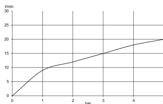
Durchflussdiagramm
