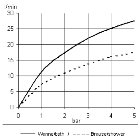
Durchflussdiagramm
