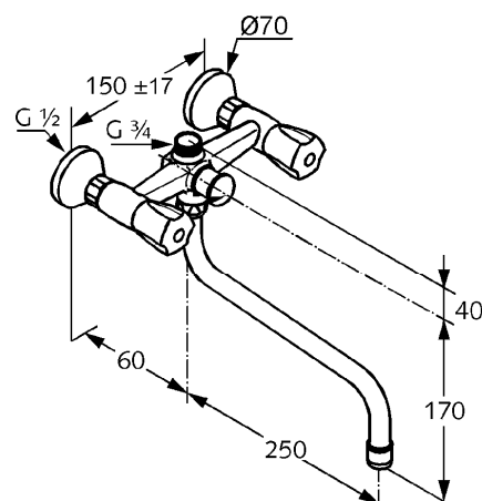
Maßzeichnung
