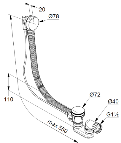
Maßzeichnung
