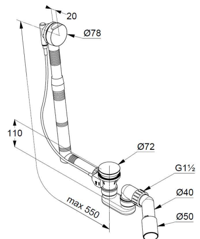
Maßzeichnung
