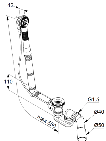
Maßzeichnung
