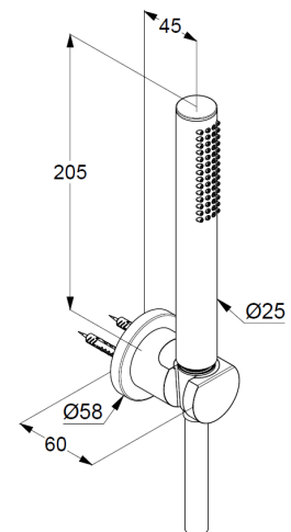
Maßzeichnung
