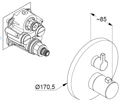
Maßzeichnung
