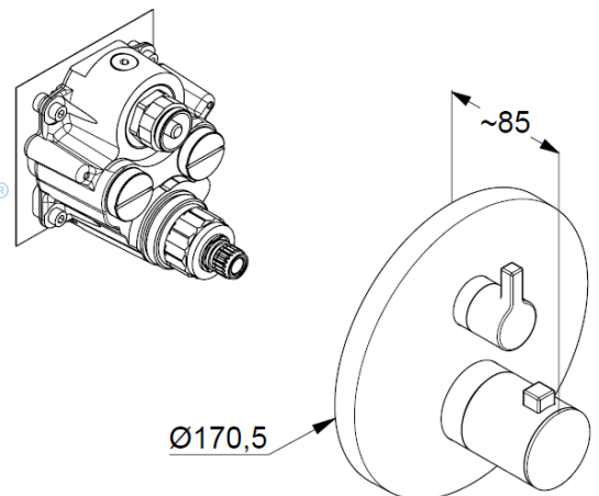
Maßzeichnung
