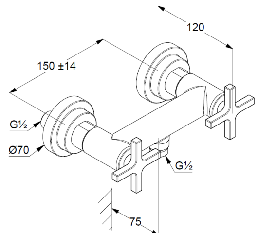
Maßzeichnung
