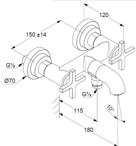
Maßzeichnung
