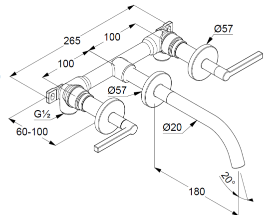
Maßzeichnung
