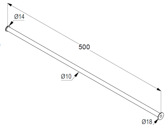
Maßzeichnung
