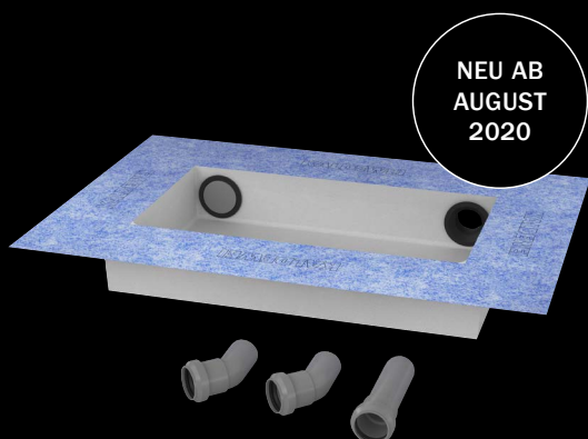
Beim Austausch von Badewanne und Duschfläche bleibt die Position der S-IX Box unverändert.
