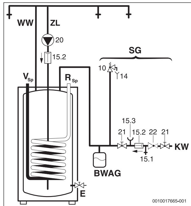
Bild 1 Trinkwasserseitiges Anschluss-Schema
